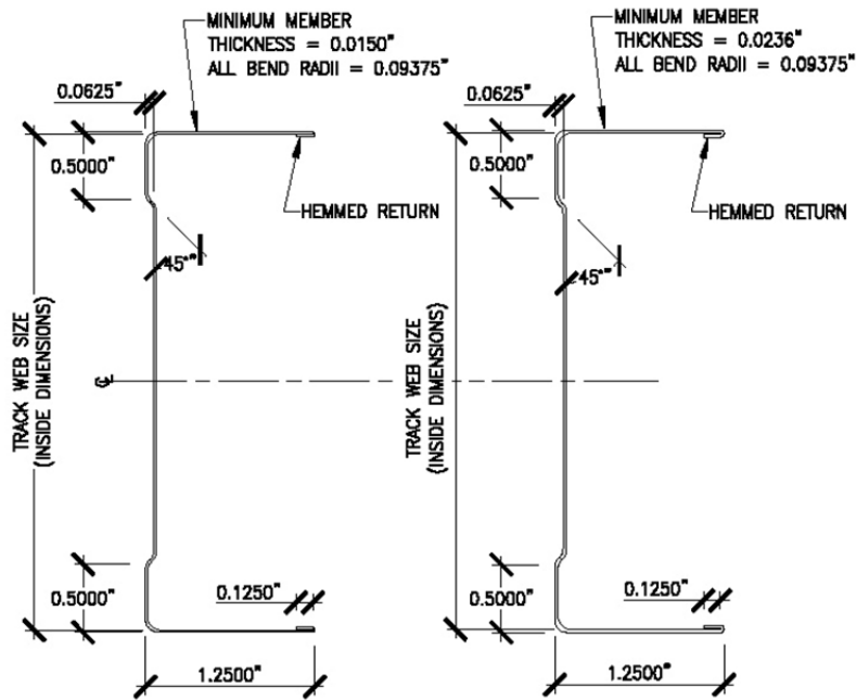
15 MIL PRIMESTUD TRACKS 24 MIL PRIMESTUD TRACKS
