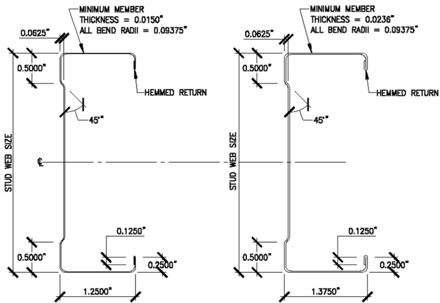
15 MIL PRIMESTUD STUDS 24 MIL PRIMESTUD STUDS
